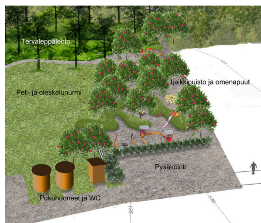
Ote Kukkonniemen ulkoilualueen yleissuunnitelmasta vuodelta 2012. Leikkipuiston nurmikumpareille on suunniteltu istutettavaksi omenapuita. Pysäköintialue on erotettu leikkipuistosta pensasistutuksin.
