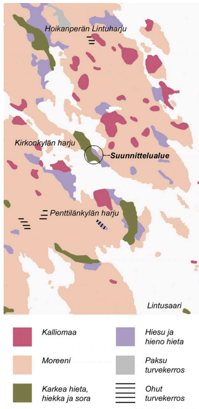
Maaperän yleiskartta (Karttalähde: GTK:n karttapalvelut 2026)
